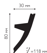
MC373 2000 x 80 x 30 мм КОМПОЗИТ
